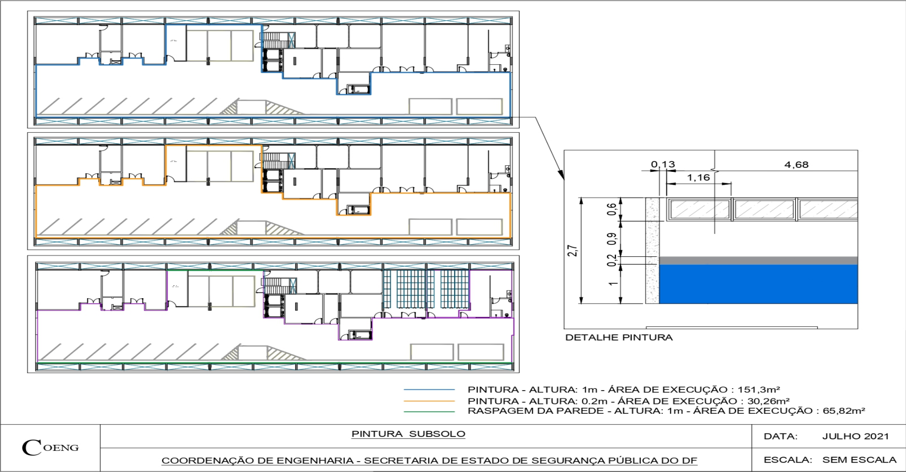
Foto 12 - Croqui de Execução de pintura das paredes da garagem
