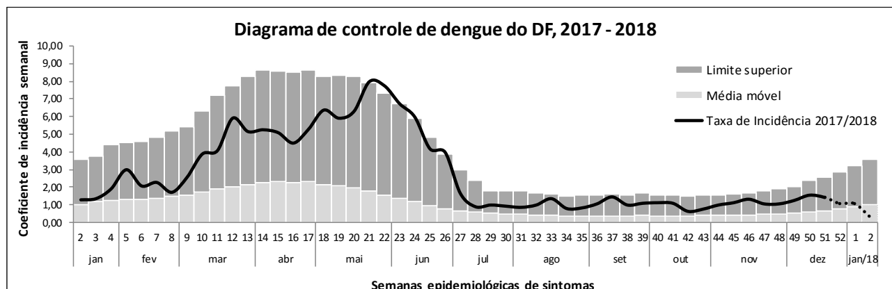
Figura 1 – Diagrama de controle e curva de incidência anual de casos prováveis de dengue em residentes do Distrito Federal, por semana epidemiológica de início de sintomas, da 2ª semana epidemiológica de 2017 até a 2ª semana epidemiológica de 2018.
